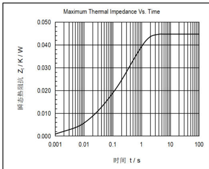
图2. 瞬态热阻抗曲线及分析曲线
